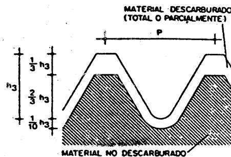
Figura 2.5.10.B Profundidad de descarburación
