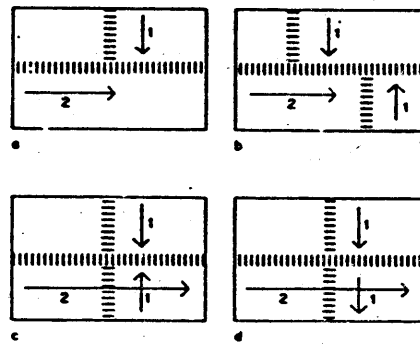
Figura 5.2.4.E Uniones planas con soldaduras que se cruzan
