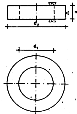
Figura 2.5.5.C Arandela pulida
