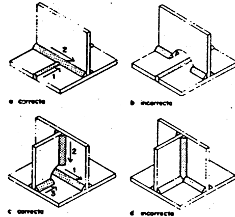
Figura 5.2.4.F Uniones en ángulo con soldaduras que se cruzan
