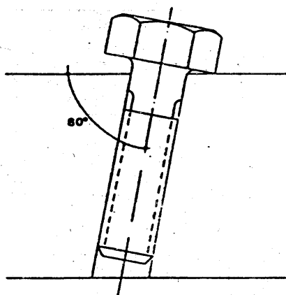
Figura 2.5.10.A Ensayo de rebatimiento
