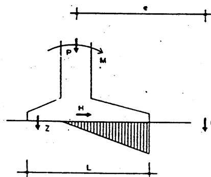
Figura 3.8.2.B Ley triangular de tensiones
