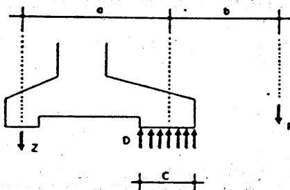
Figura 3.8.2.A Anclaje con taco de compresión
