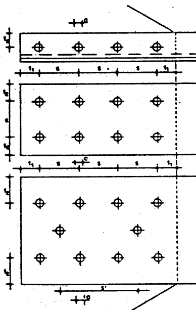
Figura 3.6.3.A Disposiciones constructivas
