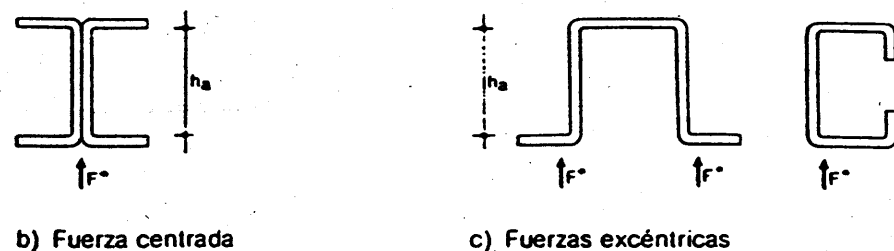
Figura 4.4.6.A Cargas concentradas (fin)
