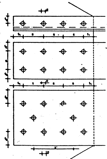
Figura 5.1.2 Separación entre agujeros
