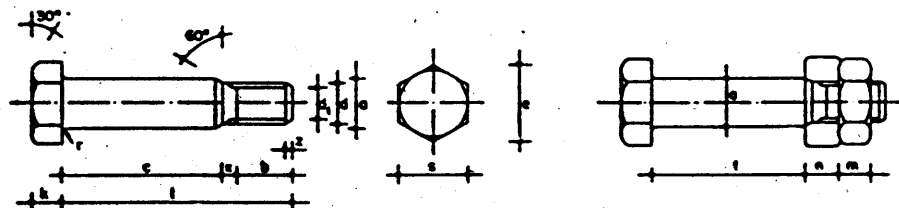
Figura 2.5.4 Tornillo calibrado
