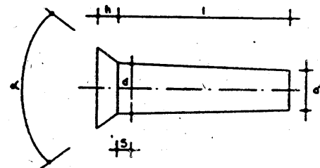
Figura 2.4.4.B Tolerancias dimensionales
