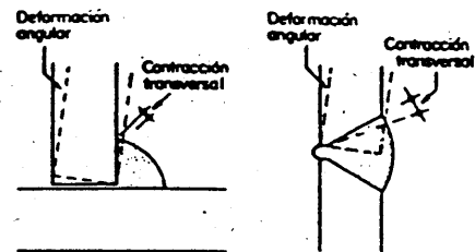
Figura 5.2.6.B Deformaciones angulares por la soldadura
