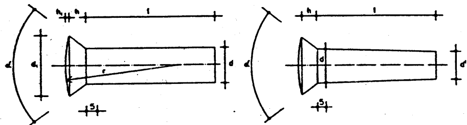
Figura 2.4.3.A Roblones de cabeza bombeada
