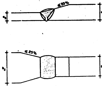
Figura 5.2.3.A Soldadura a tope en piezas de distinta sección
