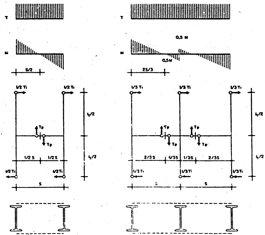
a) de dos cordones
