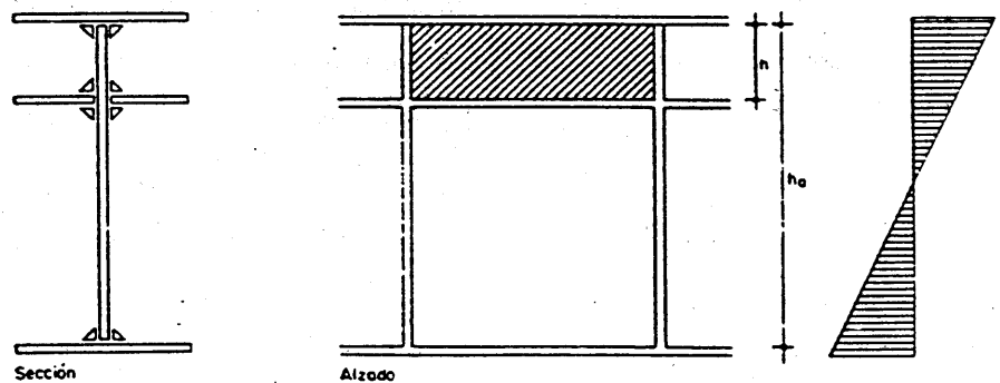
Figura 3.4.7 Rigidizadores
