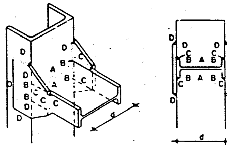
Figura 3.A6.2. Uniones espaciales con cartelas
