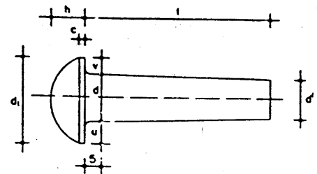
Figura 2.4.2.B Tolerancias dimensionales
