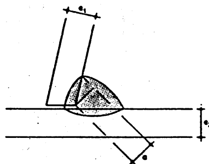
Figura 5.2.1.I Garganta a de una soldadura de ángulo
