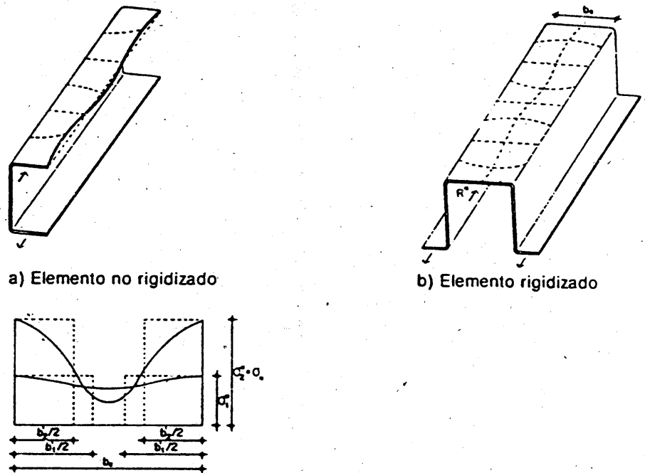
c) Tensión en el centro de las fibras a lo largo de la anchura recta b del elemento rigidizado y anchura eficaz b_1 , con \sigma_1 < \sigma_u y b_2 en agotamiento con \sigma_2 = \sigma_u
