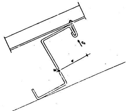
Figura 4.4.4 Correa fijada con ganchos
