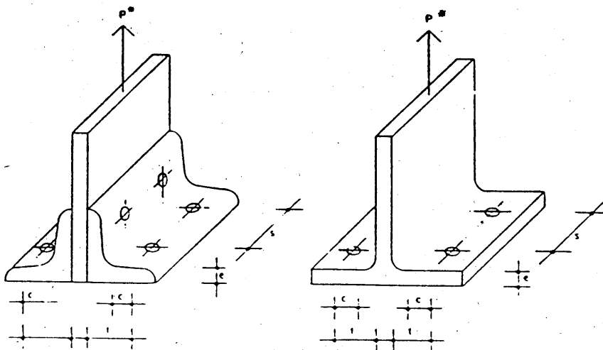
Figura 3.A5.2 Notaciones
