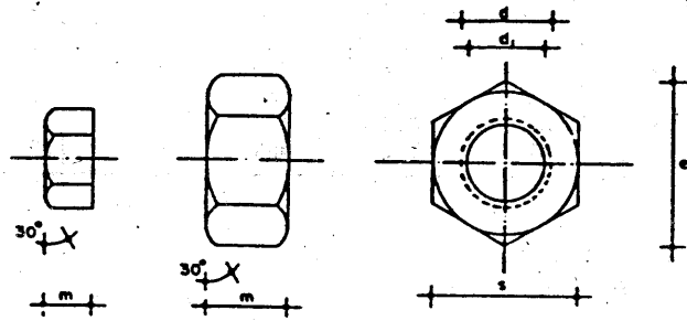
Figura 2.5.5.A Tuercas
