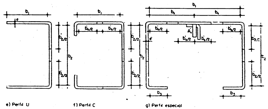
Figura 4.1.4 Secciones eficaces de perfiles sometidos a flexion simple (casos a, b, c y d) y a compresión (casos e, f y g)
