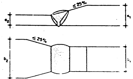
Figura 3.7.2 A Soldadura a tope de chapas de distinta sección
