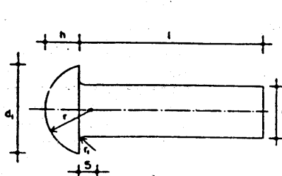
Figura 2.4.2.A Roblones de cabeza esférica
