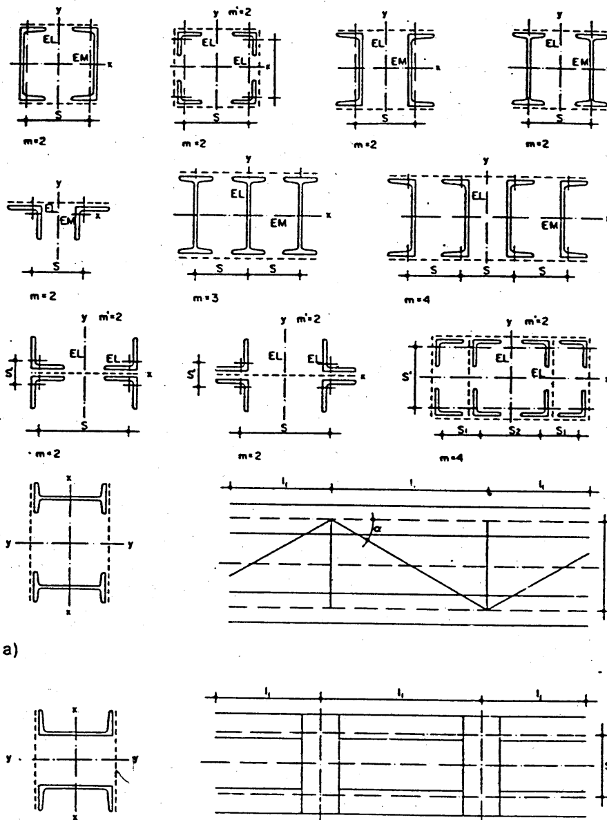
Figura 3.2.5.2 Secciones de piezas compuestas
