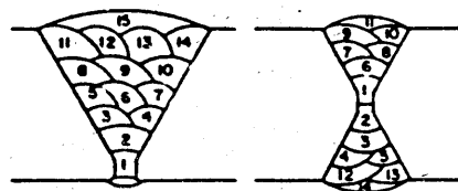
Figura 5.2.4.A Soldadura de varios cordones
