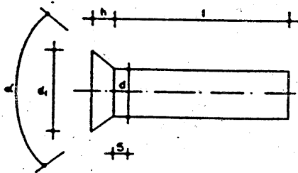
Figura 2.4.4.A Roblones de cabeza plana
