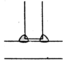
Figura 5.2.1.D Soldadura de ángulo en rincón
