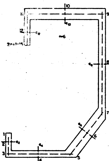
Figura 4.A1.1 Sección abierta poligonal de tramos
