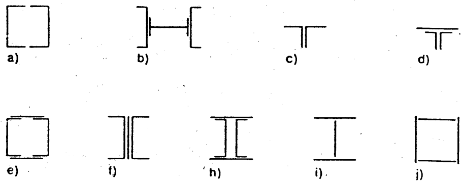
Figura 3.2.1.1.A Esquemas de piezas simples constituidas por perfiles o chapas yuxtapuestas
