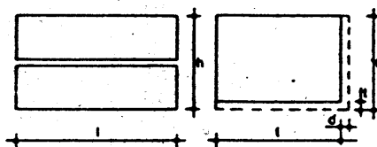
Figura 5.2.6.A Deformaciones lineales por la soldadura
