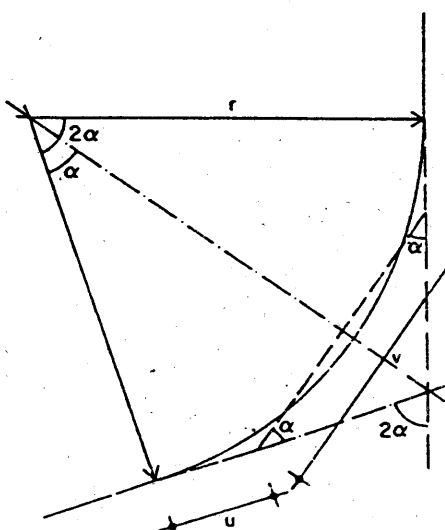
Figura 4.A1.3 Sustitución de un acuerdo curvo por uno quebrado
