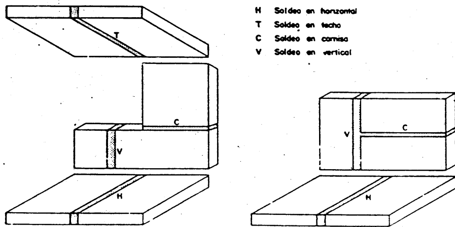
Figura 5.2.7 Posiciones de soldeo
