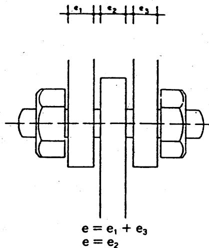
Figura 3.8.2.D Unión de chapas con pasador
