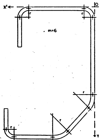
Figura 4.A1.2 Sección de una pieza de chapa conformada
